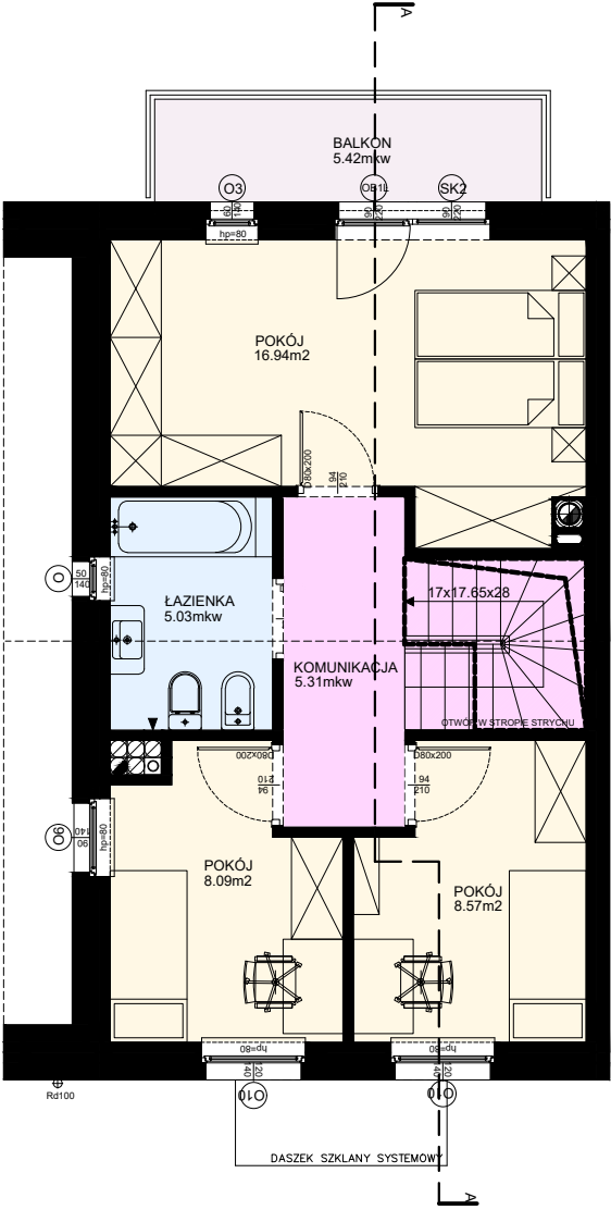
PODDASZE
