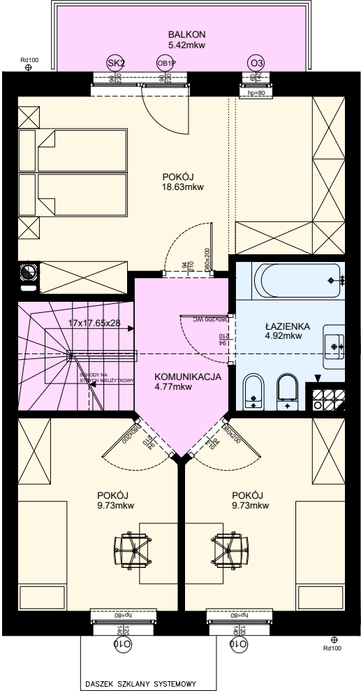
PODDASZE
