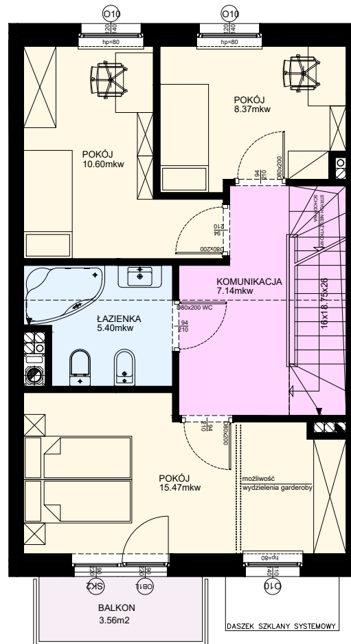
PODDASZE
